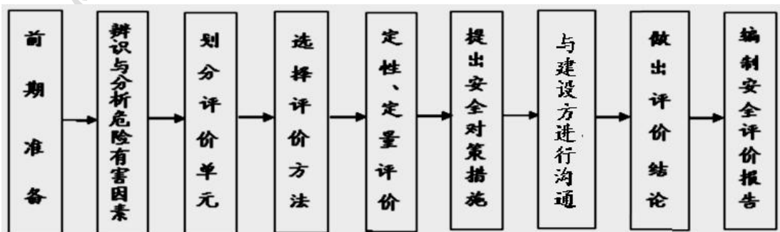
图 1-1 安全现状评价程序框图
